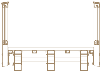
Frontansicht
