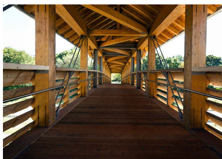
Innenansicht
