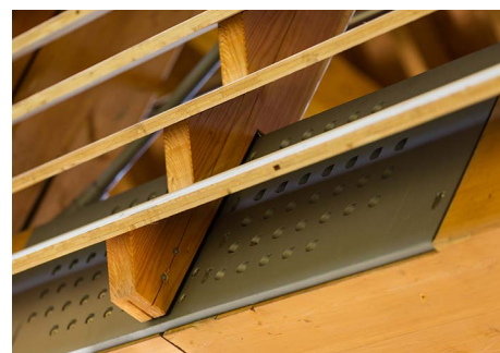
Lamellen-Verschalung
